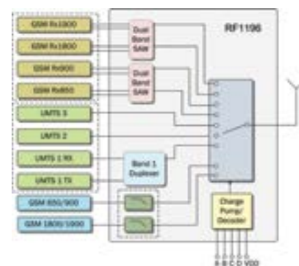
Switch Duplexer Module
